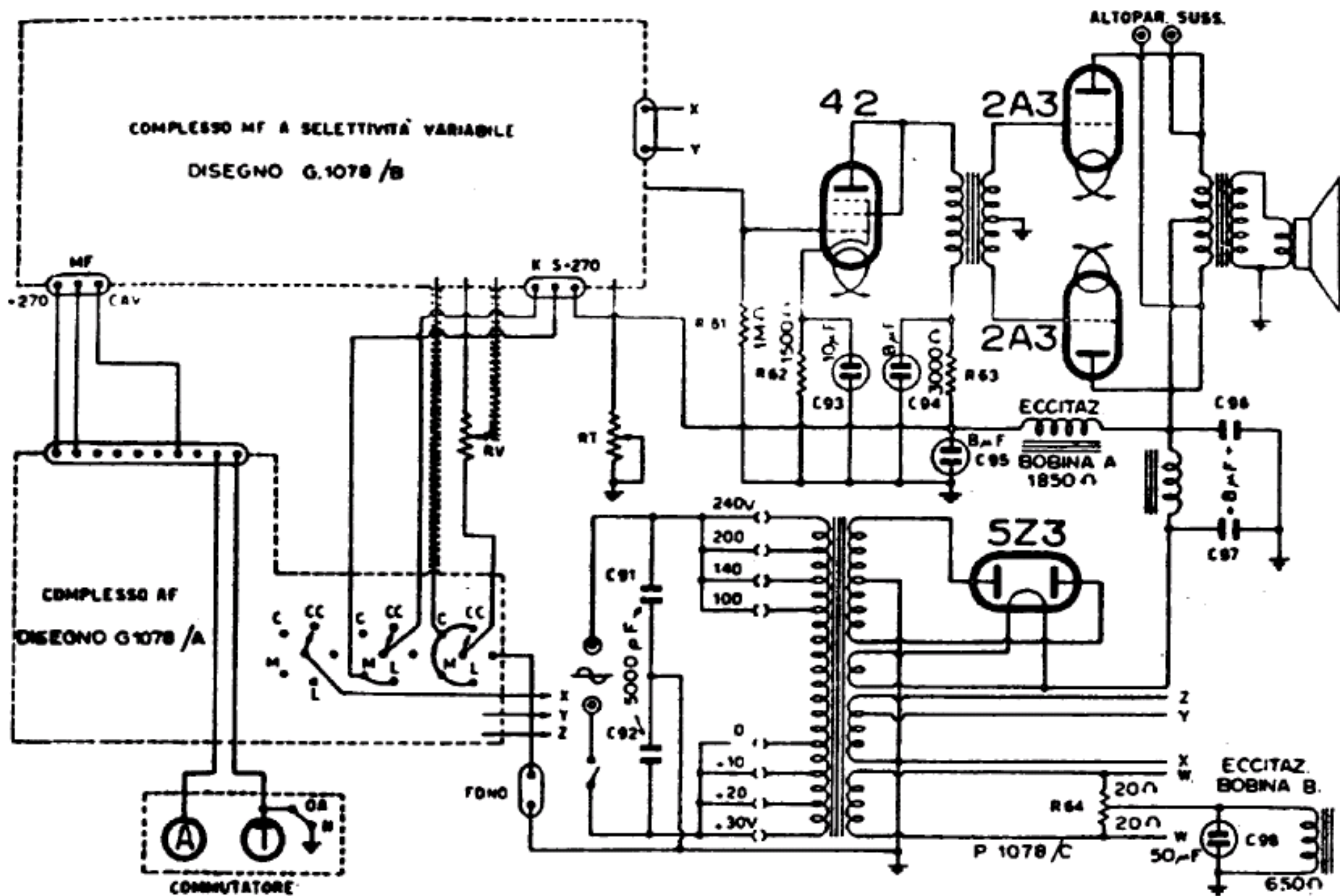
F.I.M.I. - MOD. PHONOLA « 880 » - PARTE BF
